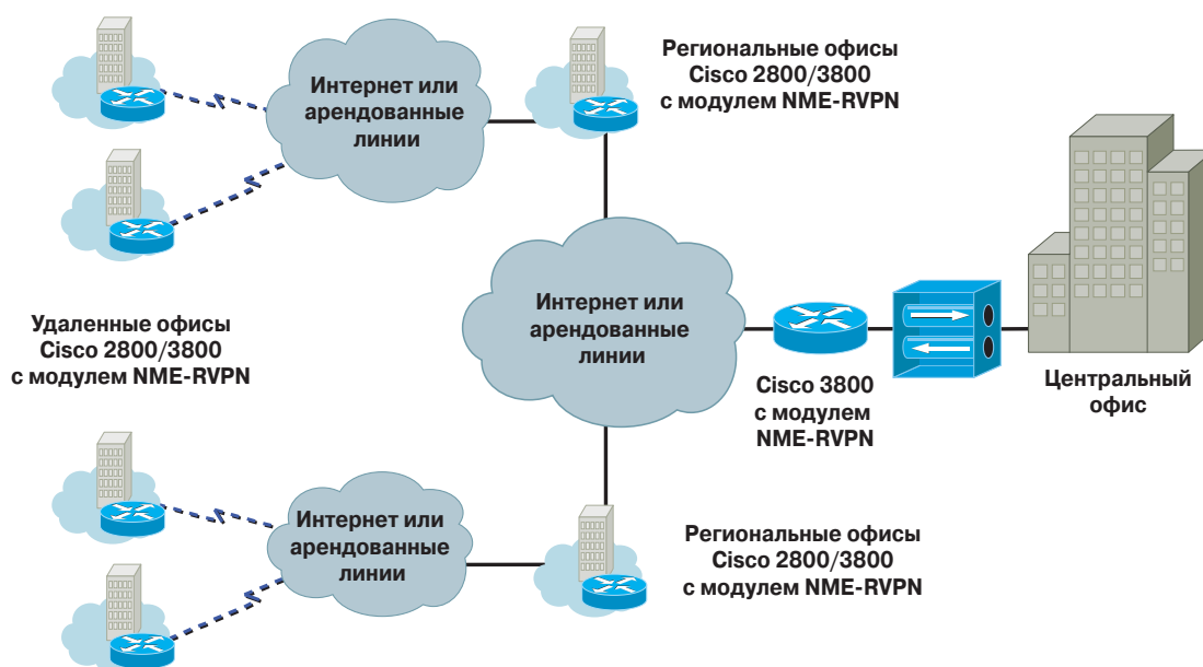
Рисунок 2. Использование VPN-туннелей для создания защищенной корпоративной сети
